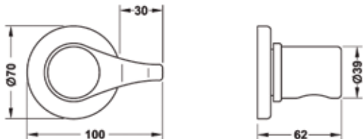
gałka obrotowa
