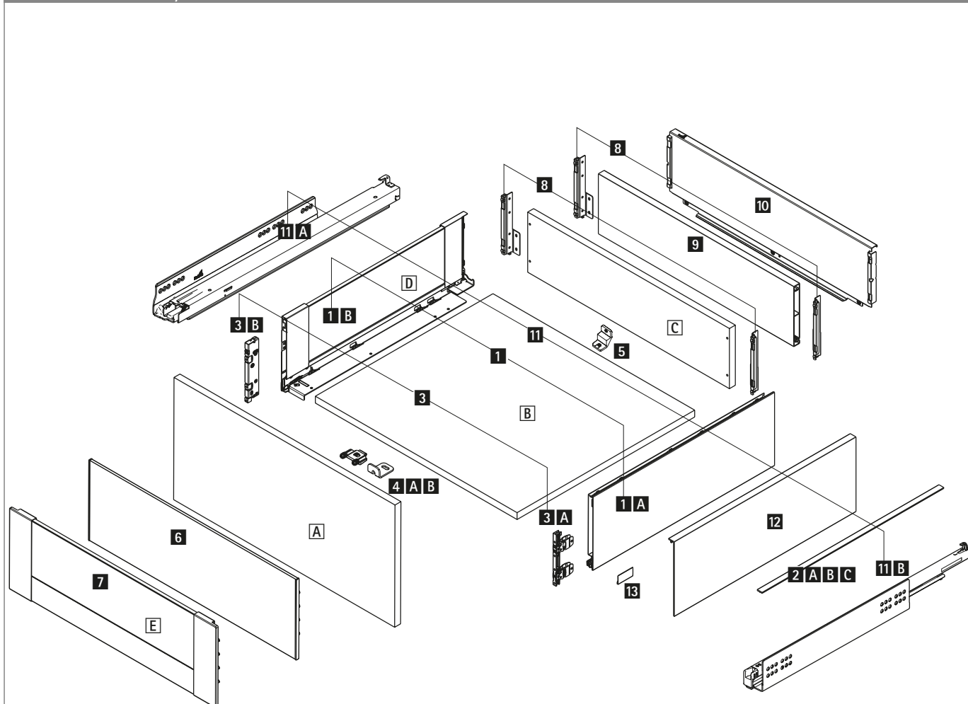
Widok rozstrzelony
