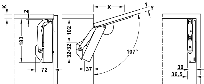
Wymiary
