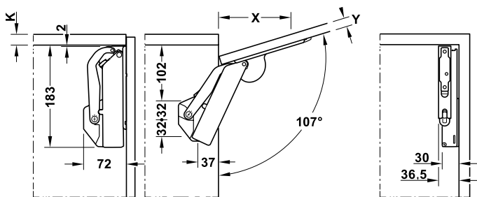
Wymiary
